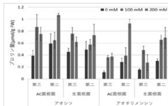
生重量あたりのプロリン量(図1)(n=3, 標準誤差)
