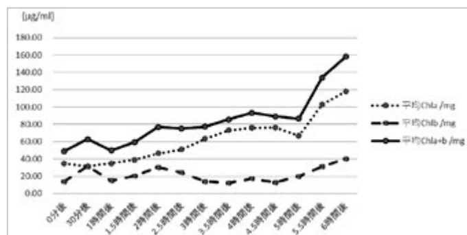
図 1 照射時間によるクロロフィル量の変化
