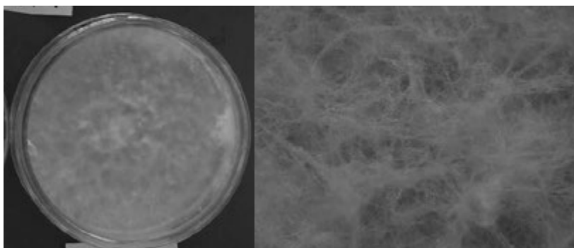
写真. UV40分照射で生じた孢子形成能力欠損突然変異株 左：培養6日目シャーレの様子 右：実体顕微鏡検鏡下の菌糸
