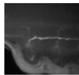
蛍光顕微鏡による観察 (実験5)
