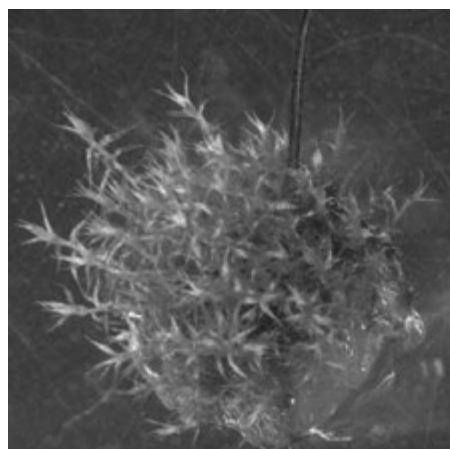
図.胞子体殺菌実験で得られた無菌の配偶体の様子
