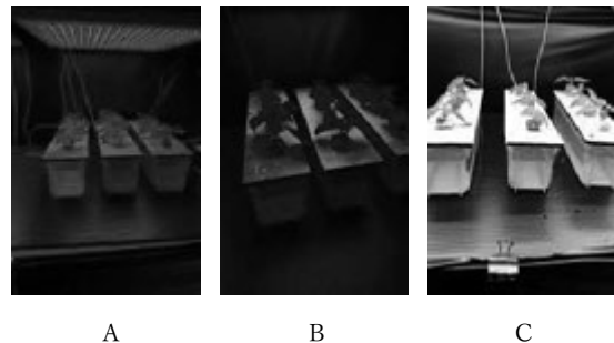
図1 各光環境下での栽培の様子 A:赤色 LED B:赤色 LED C:蛍光灯
