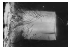
子房切片への誘引（アニリンブルー染色）
