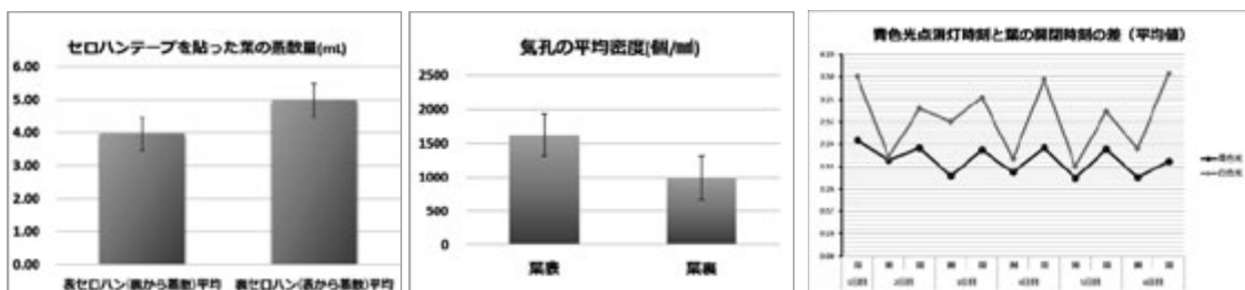
図1 葉の表裏の蒸散量
