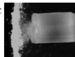
寒天に埋めた子房切片
