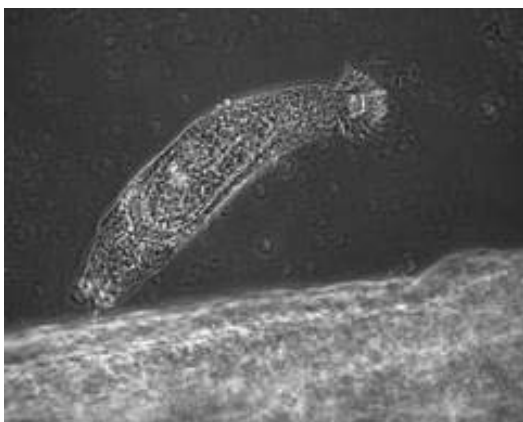
図1 色素で薬浴すると、宿主から脱落した寄生虫・ギロダクチルス（位相差顕微鏡で撮影、対物 x10）
